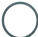
80093 D1= \Phi 70mm D2= \Phi 82.5mm Height= 4.7mm OEM: 9091706031
