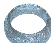
80440 D1= \Phi 35mm D2= \Phi 46mm Height= 15.1mm OEM: 174510Q010
