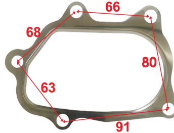
G-SUB-1 S/Steel Fits FL-SUB / Subaru Impreza
