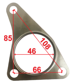
G-SUB-2 S/Steel Subaru Impreza
