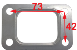
G-T25 S/Steel Fits FL-T25
